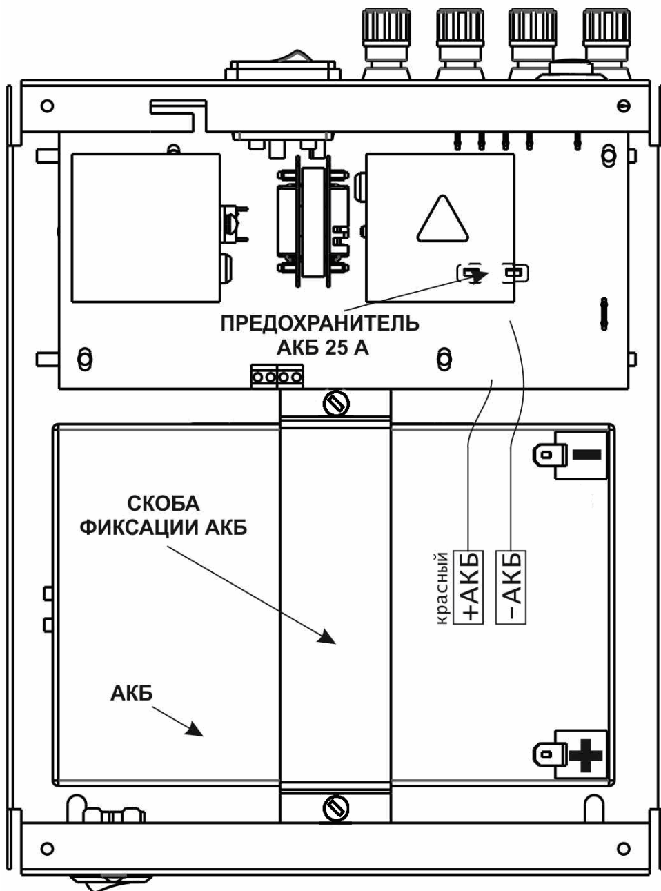
Рис.3 Расположение коммутационных элементов ВОЛНА ББП – 3/20 при снятой крышке корпуса ФИАШ.436234.434 РЭ-4 Формат А5 9
