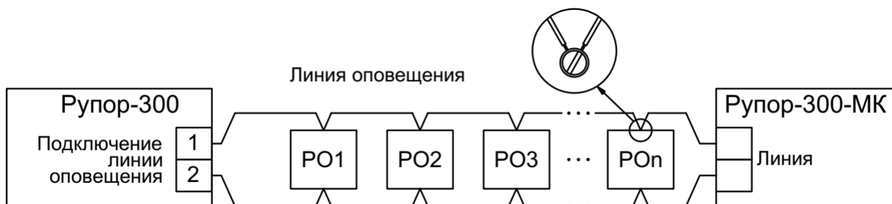
Рисунок 2. Подключение модуля Рупор-300-МК.
