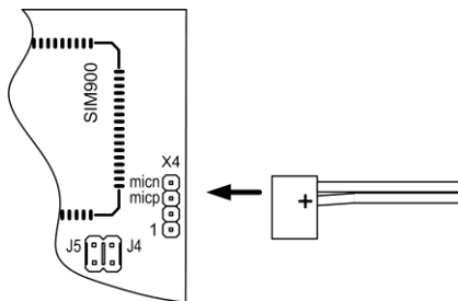
Рисунок 15.3 – Подключение микрофона к коммуникатору
