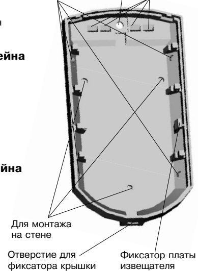
Рисунок 2 – Основание извещателя и кронштейн
