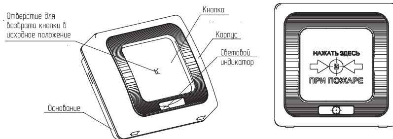
Рисунок 1- Внешний вид и устройство извещателя
