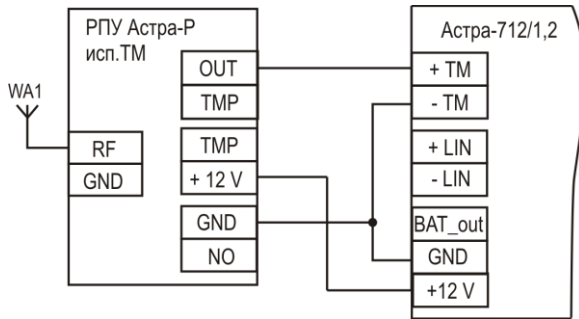
Рисунок А.1- Схема подключения «РПУ Астра-Р» исполнения ТМ
