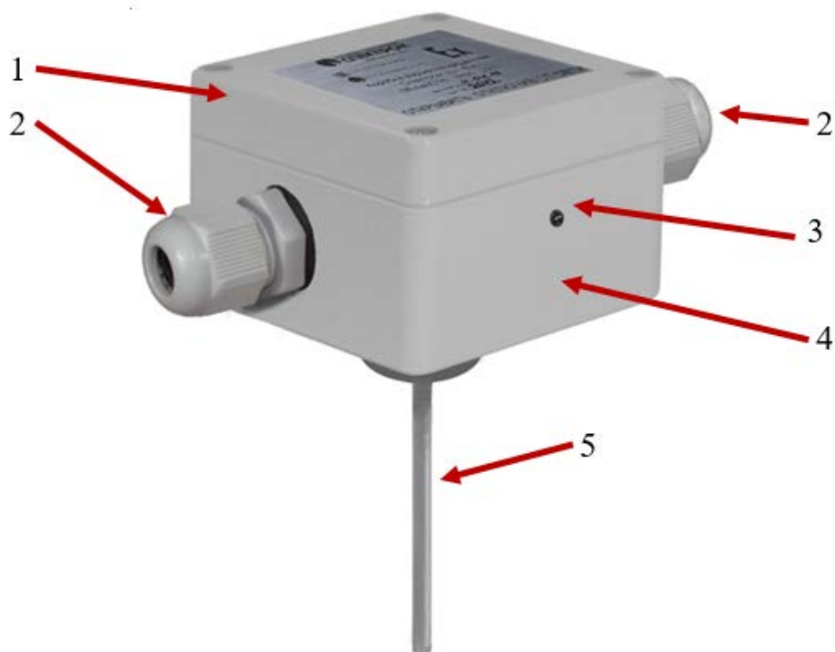
Рис.3 – Внешний вид извещателя
