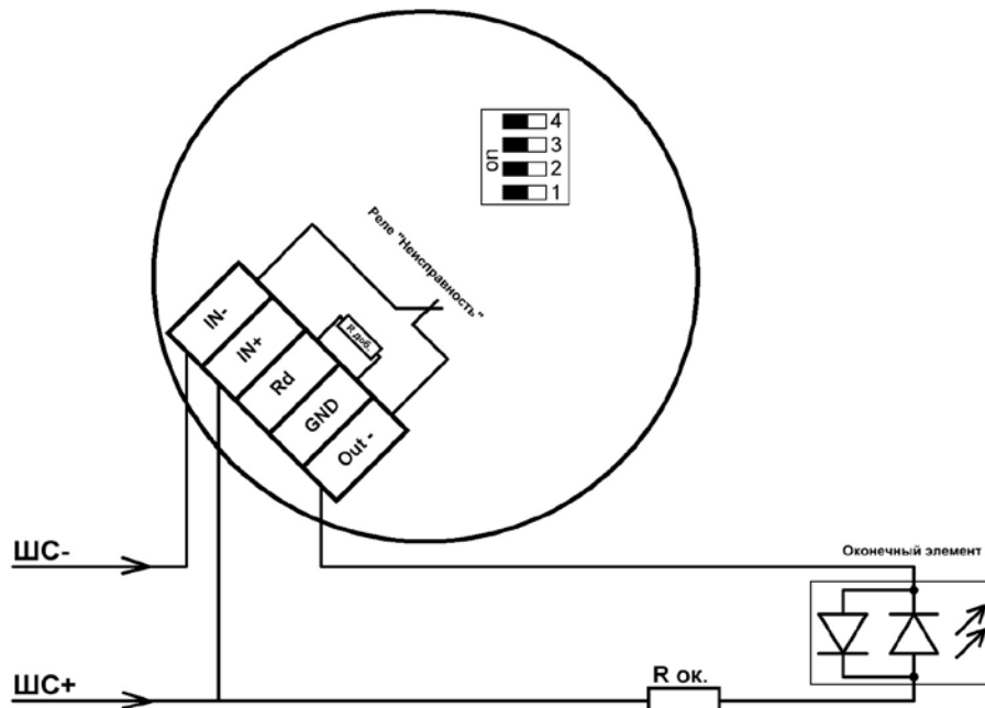
Рисунок 4 – Подключения по 2-х проводной схеме с режимом «Неисправность»
