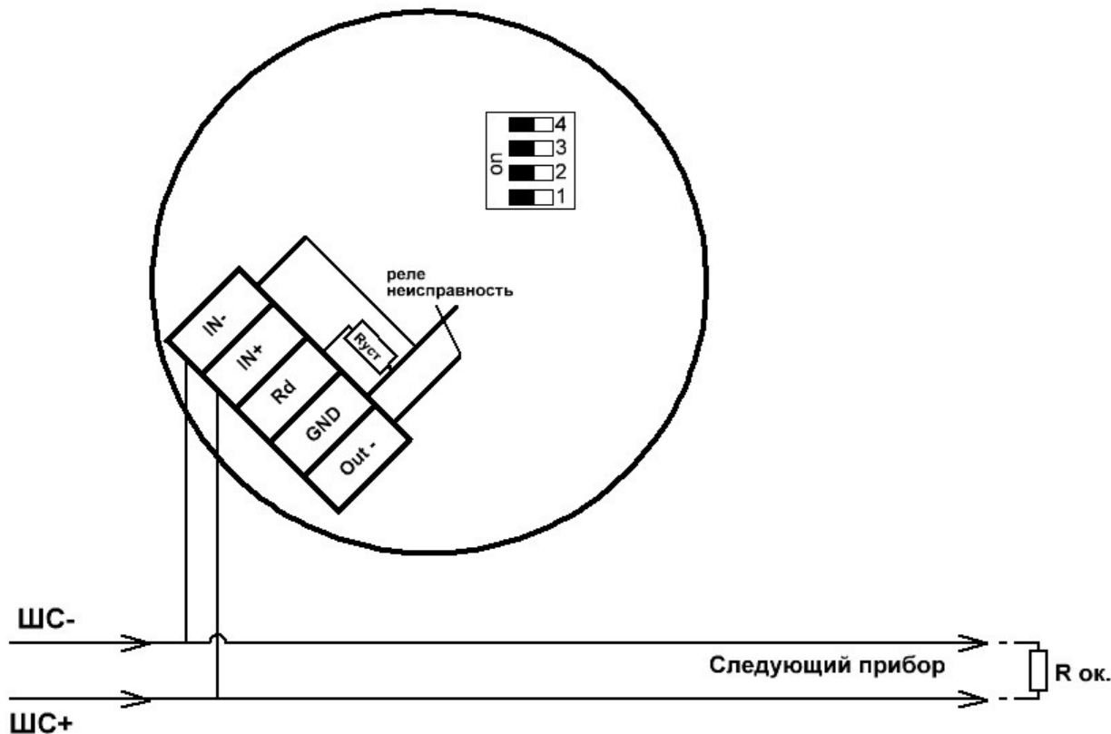
Рисунок 5 – Подключение по 2-х проводной схеме без режима «Неисправность»
