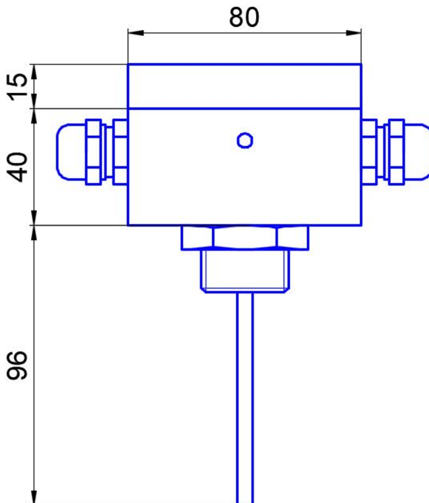
Рис. 1 – Извещатель пожарный тепловой Спектрон-101-Р-Ехi/Ехm
