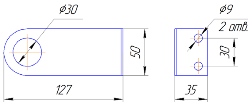
Рис. 2 – Крепежное устройство (Спектрон-К-05 серого цвета)
