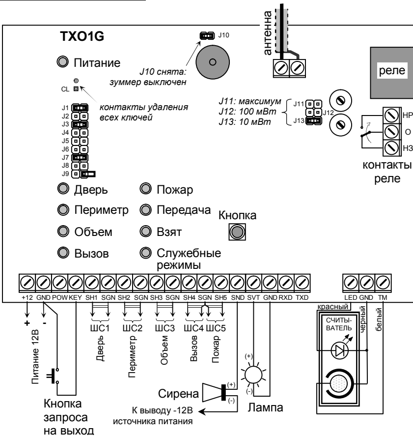
Рисунок 6 – Монтажная схема передатчика
