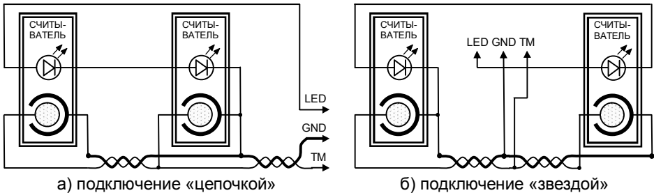
Рисунок 4 – Подключение двух считывателей
