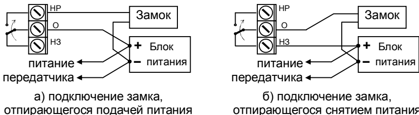
Рисунок 5 – Подключение электрического замка
