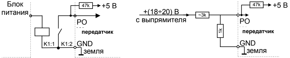
а) выход БП – реле на землю
