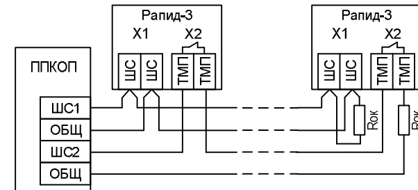
Рис.2 Схема подключения извещателей к ППКОП
