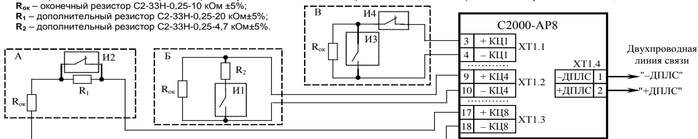
Рисунок 1 Схема соединений
