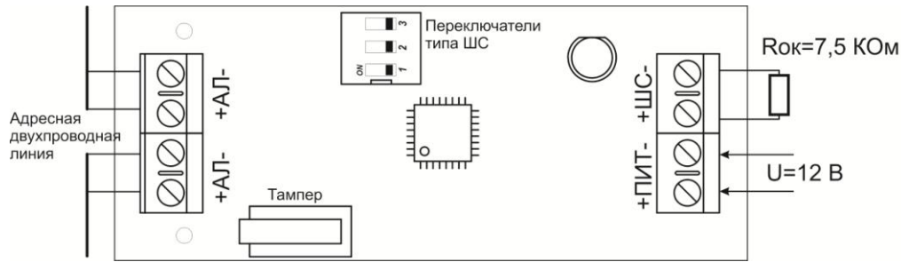
Рис. 1 Схема подключения адресной метки.
