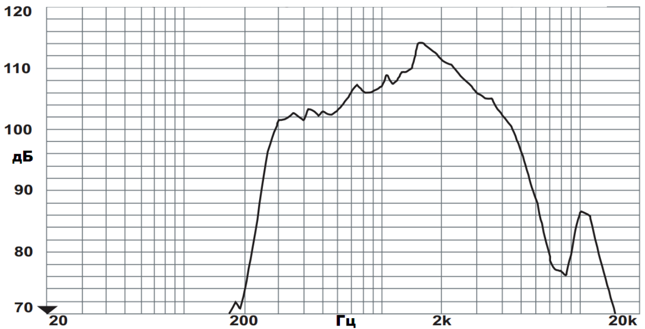
Рисунок 8 – Диаграмма направленности и амплитудно-частотная характеристика ГВР-Ехd-30
