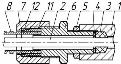
монтаж кабелем в металлорукаве KB15
