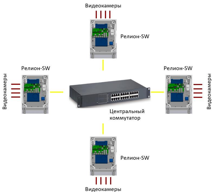
Рисунок 8. Подключение коммутаторов в топологию «звезда»
