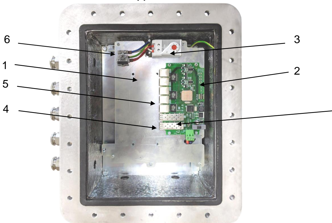
Рис. 5. Расположение составных частей Релион-SW-M-2G-4Poe+/240W 1- Источник питания; 2- Индикаторы состояния портов коммутатора; 3- термостат; 4- SFP 100/1000 Base-FX порт коммутатора; 5- 10/100 Base-TX порты коммутатора с поддержкой PoE; 6- предохранитель.
