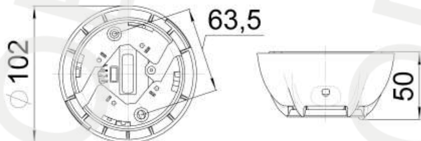
Рисунок 2 – Монтажная схема
