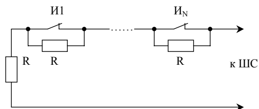
Подключение в ШС тепловых извещателей
