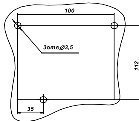
Разметка для установки прибора
