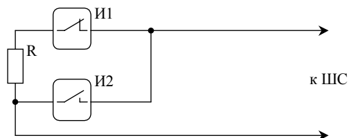
Подключение ШС в охранном режиме
