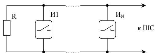
Подключение в ШС дымовых извещателей
