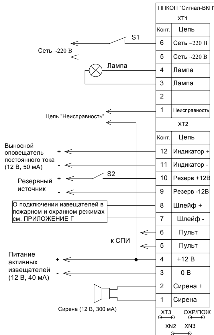
Схема электрическая соединений прибора
