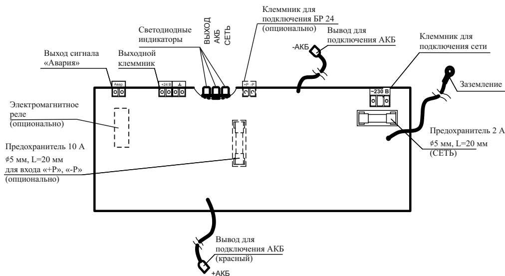
Рисунок 1 – Плата источника
