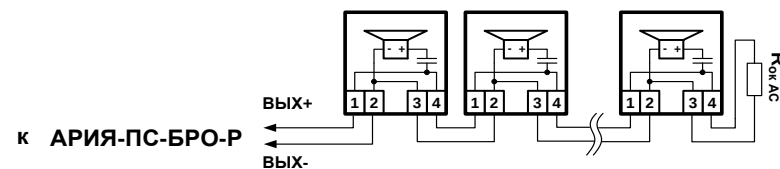
Рис. 1А. Схема соединений 1, 2, 3 и 4 речевых оповещателей серии АРИЯ-ПС.
