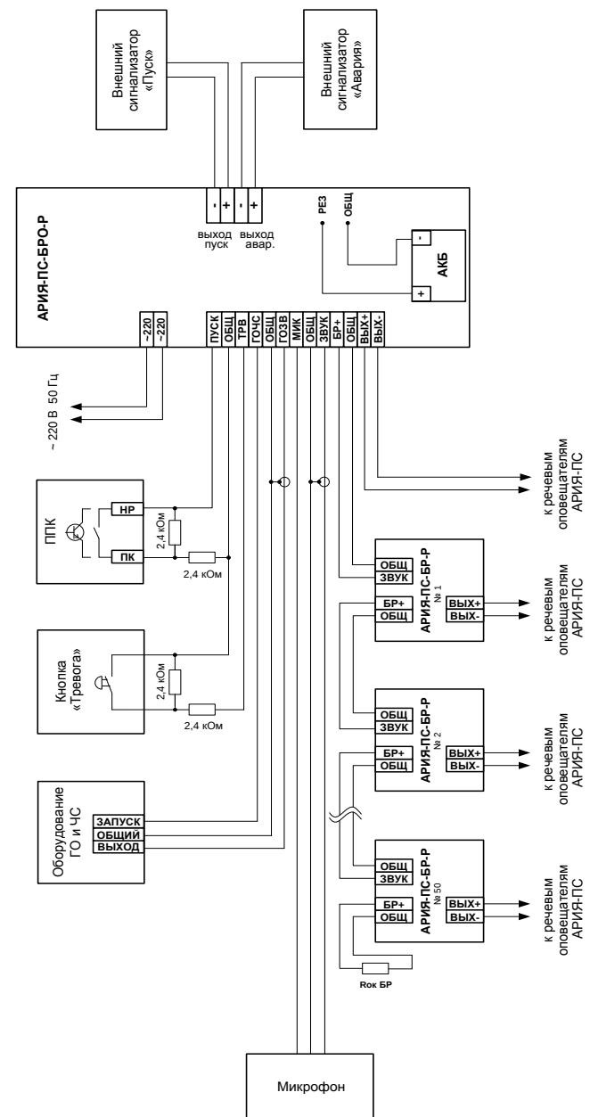
Рис. 2. Схема соединений блока речевого оповещения АРИЯ-ПС-БРО-Р
