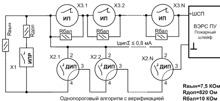
Рисунок Б4. Комбинированная схема включения ШСП.
