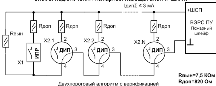
Рисунок Б2. Схема включения ШСП типа ШННС и ШПНС с несколькими дымовыми извещателями (типа ИП212).
