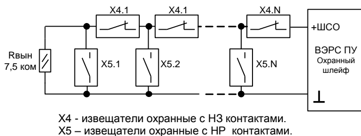
Рисунок Б6. Схема включения охранных извещателей в ШСО.
