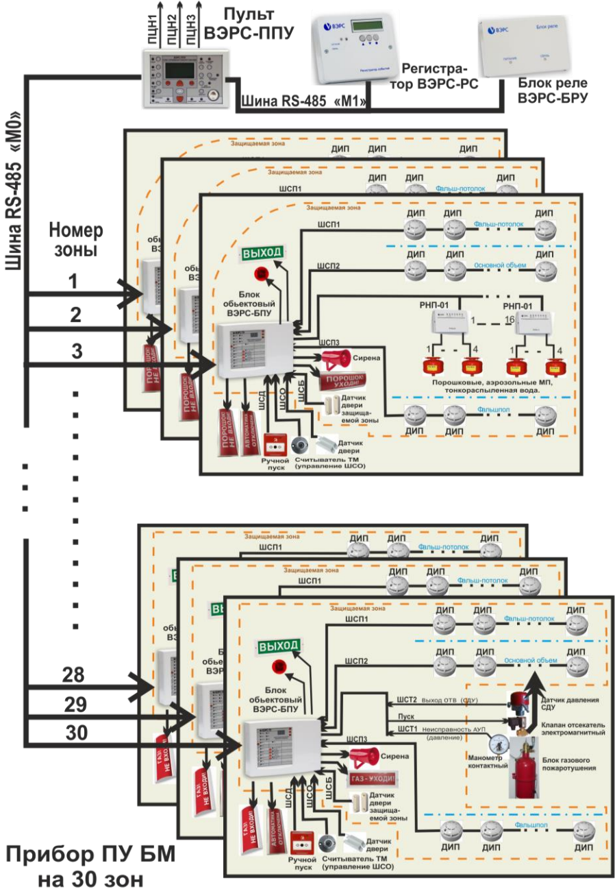
Рисунок В1. Структура автоматической системы противопожарной защиты, выполненной на ВЭРС-ПУ БМ.
